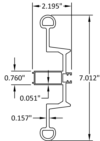
16 ASTRAGAL STILE
