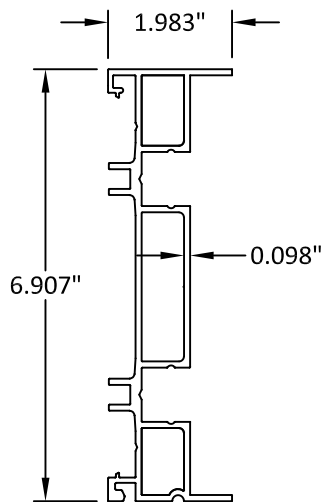
12 2 TRACK FRAME JAMB
