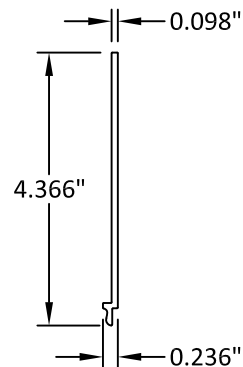
9 SILL RISER
